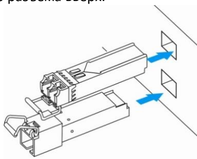
Рисунок 53 – Установка SFP-трансиверов
