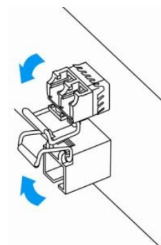
Рисунок 55 – Открытие защелки SFP-трансиверов
