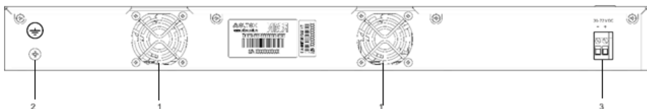
Рисунок 33 – Задняя панель MES2448 DC
