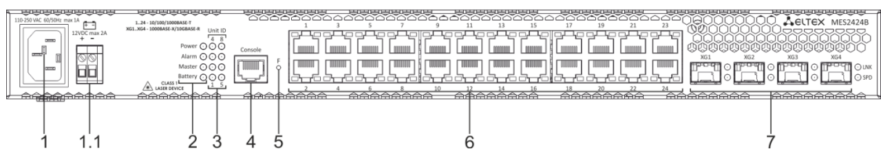
Рисунок 18 – Передняя панель MES2424В
