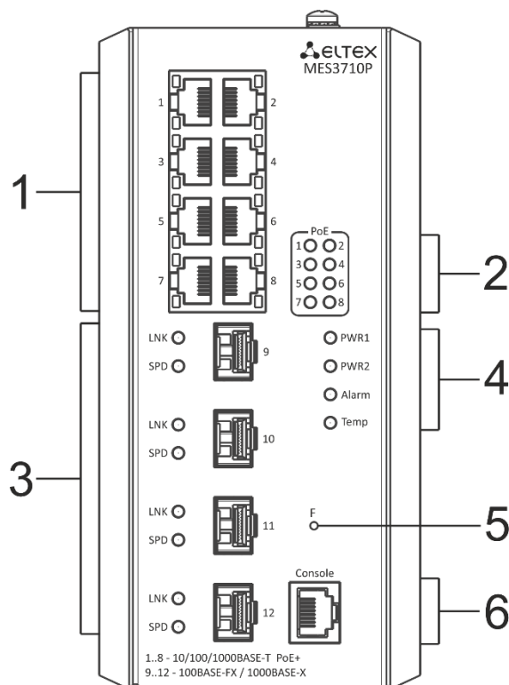
Рисунок 29 – Передняя панель MES3710P
